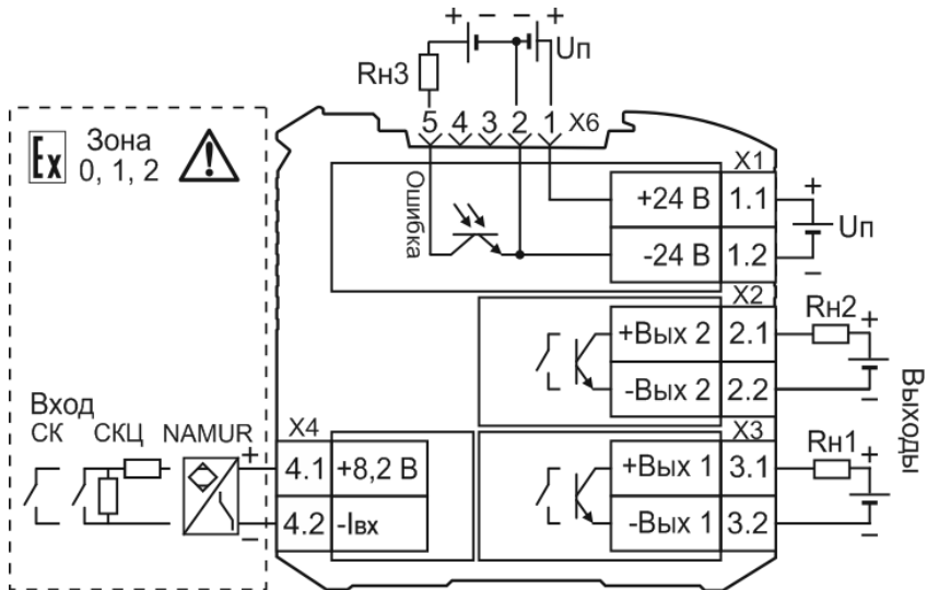
Рисунок 6.3 – Типовые схемы подключения барьеров KA5241Ex-NN
