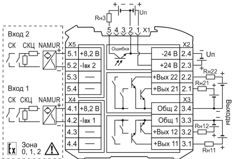
Рисунок 6.5 – Типовые схемы подключения барьеров KA5262Ex-NN
