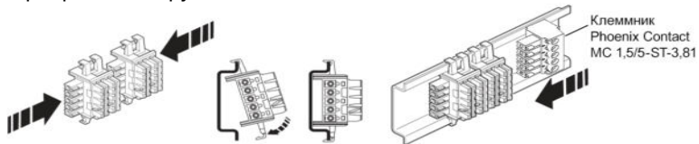
Рисунок 6.6 – Установка шинных соединителей на DIN- рейку
