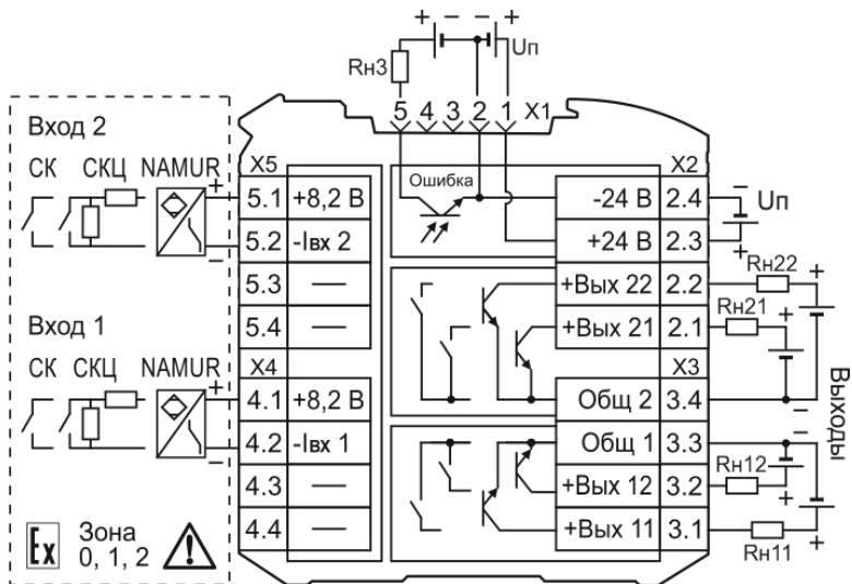
Рисунок 6.4 – Типовые схемы подключения барьеров KA5242Ex-NN
