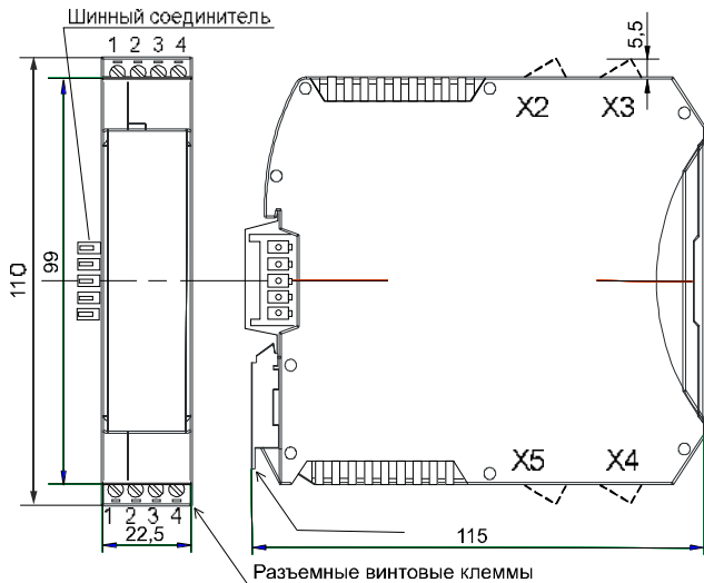
Рисунок 6.2 – Габаритные размеры барьера КА5242Ех-NN, КА5262Ех-NN
