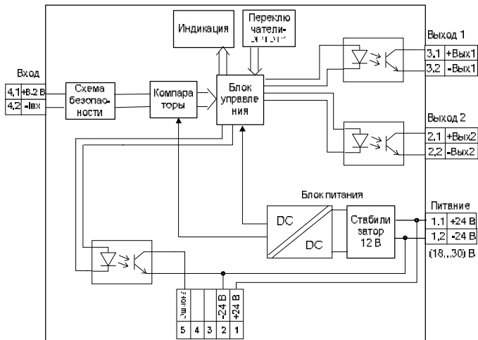
Рисунок 5.2 – Функциональная схема барьера KA5241Ex-12
