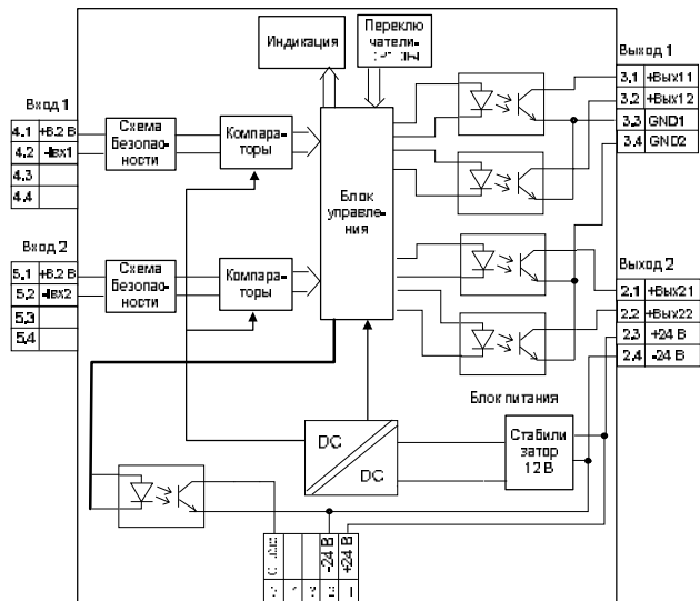
Рисунок 5.3 – Функциональная схема барьера KA5242Ex-12
