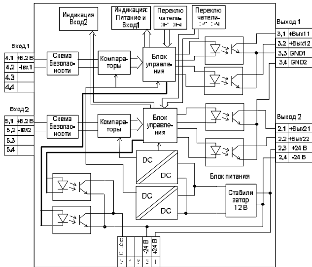
Рисунок 5.4 – Функциональная схема барьера KA5262Ex-12
