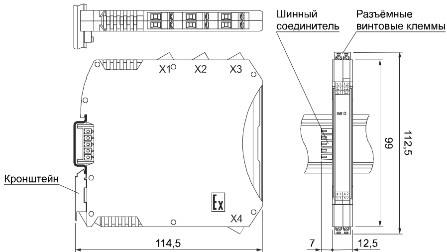
Рисунок 6.1 – Габаритные размеры барьера КА5241Ex-NN
